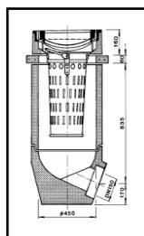
LOVILNIK NEČISTOČ
