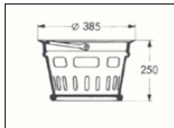
LOVILNIK NEČISTOČ
